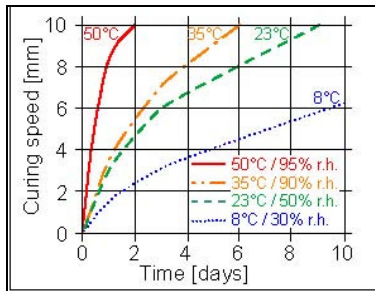
Diagrama 1: Velocidad de curado 1-C-Sikasil®
